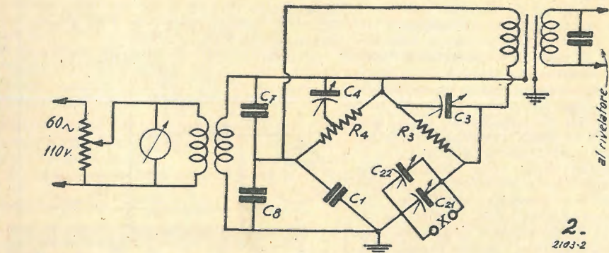
fig. 2 - Circuito del ponte di Schering per la minore portata del fattore di perdita D_x .
